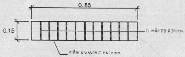
แบบขยายเหล็กตะแกรงกรองเศษขยะ ปรับปรุงทางเท้า คสล.
