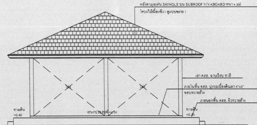
รูปด้าน 2 SCALE 1 : 75
