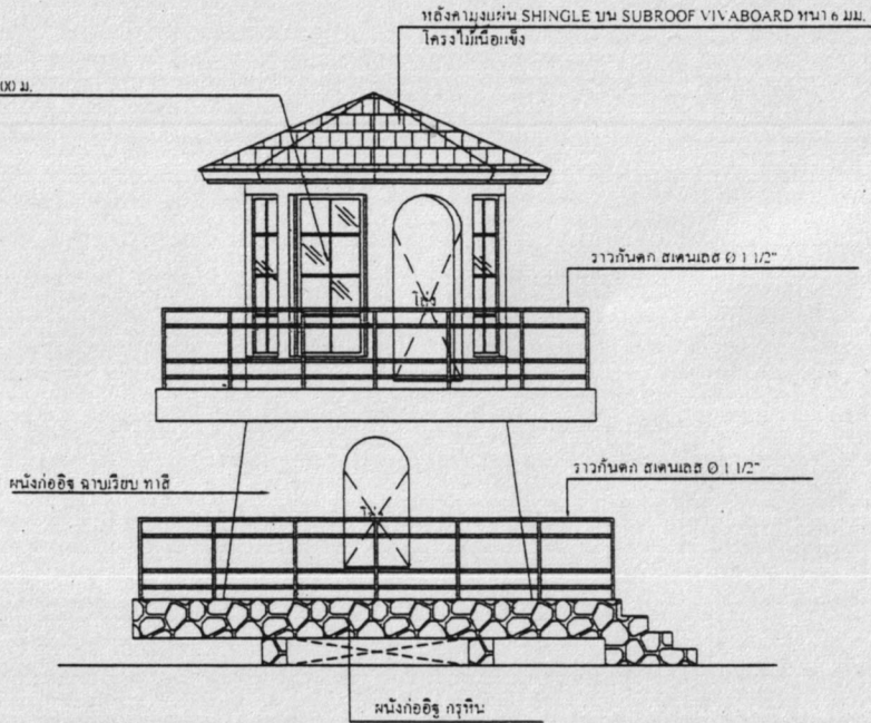
รูปด้าน 4 SCALE 1 : 75
