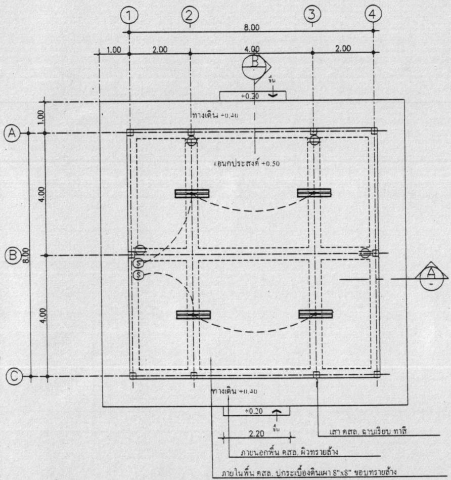
แปลนพื้น SCALE 1 : 100
