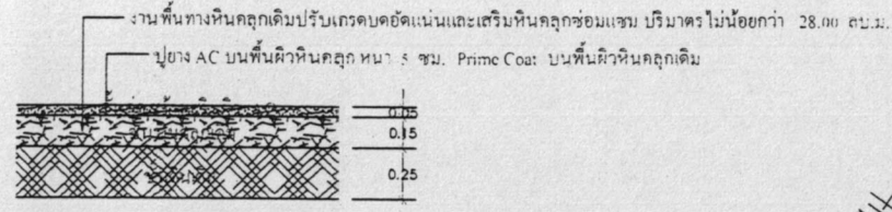
แบบแสดงรายละเอียดโครงสร้างพื้นลานจอดรถ
