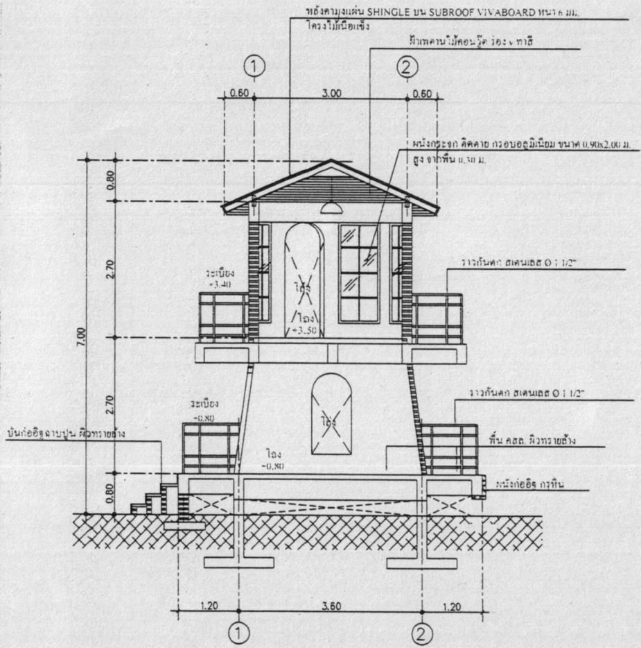
รูปตัด A SCALE 1 : 25
