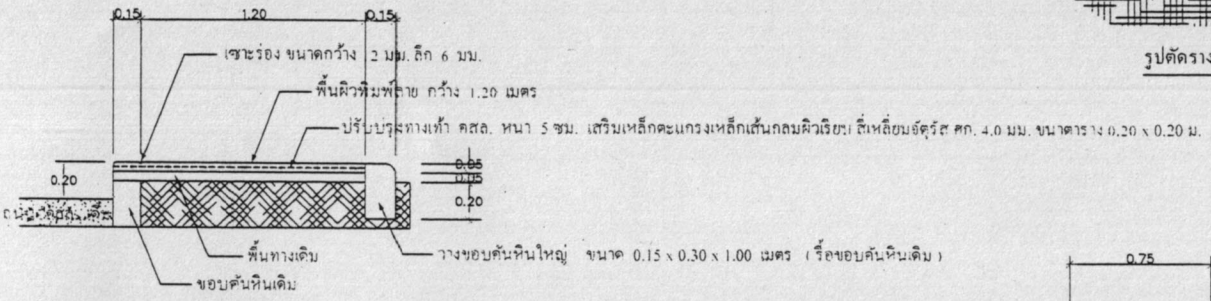
รูปตัดปรับปรุงทางเท้า คสล.
