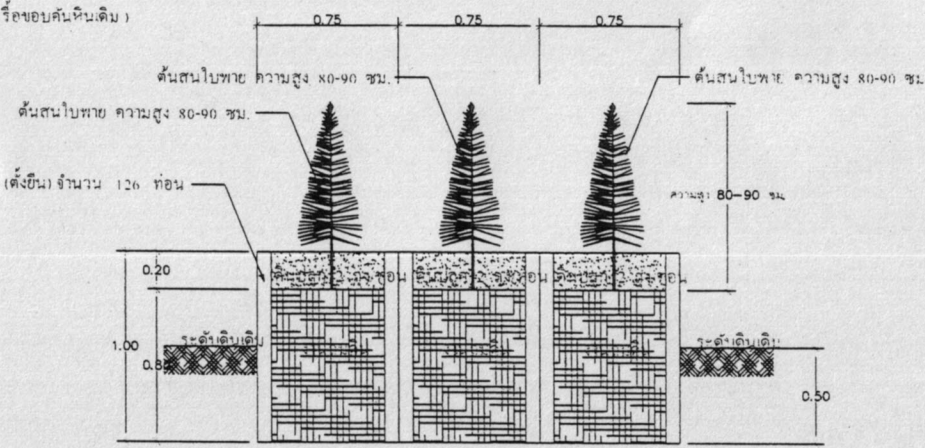
รูปตัดท่อระบาย คสล. (ตั้งหิน)
