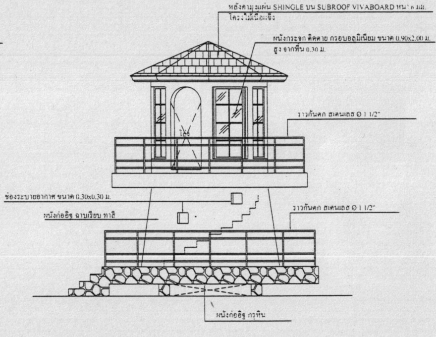
รูปด้าน 2 SCALE 1 : 75
