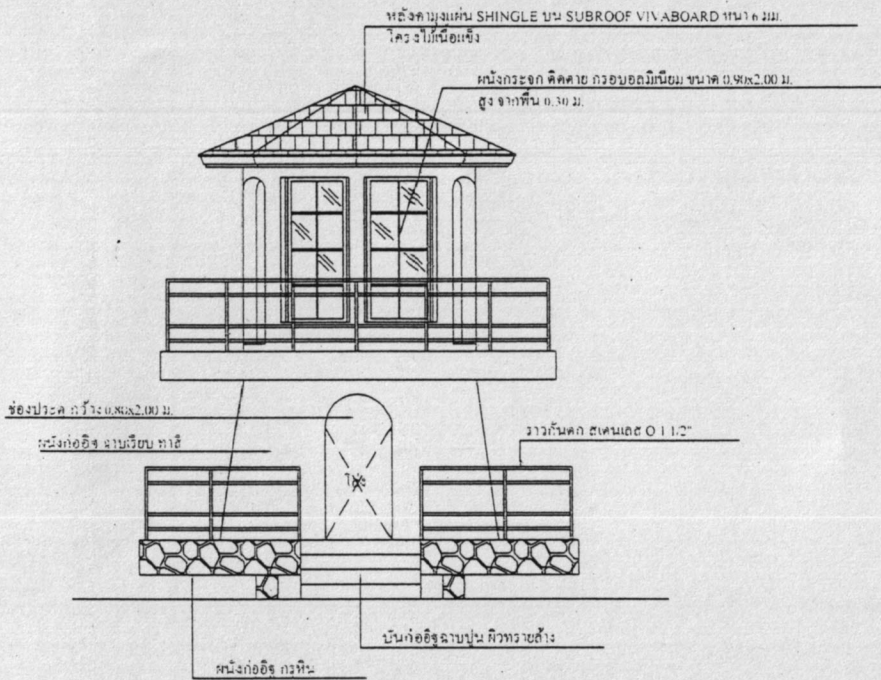
รูปด้าน 1 SCALE 1 : 75
