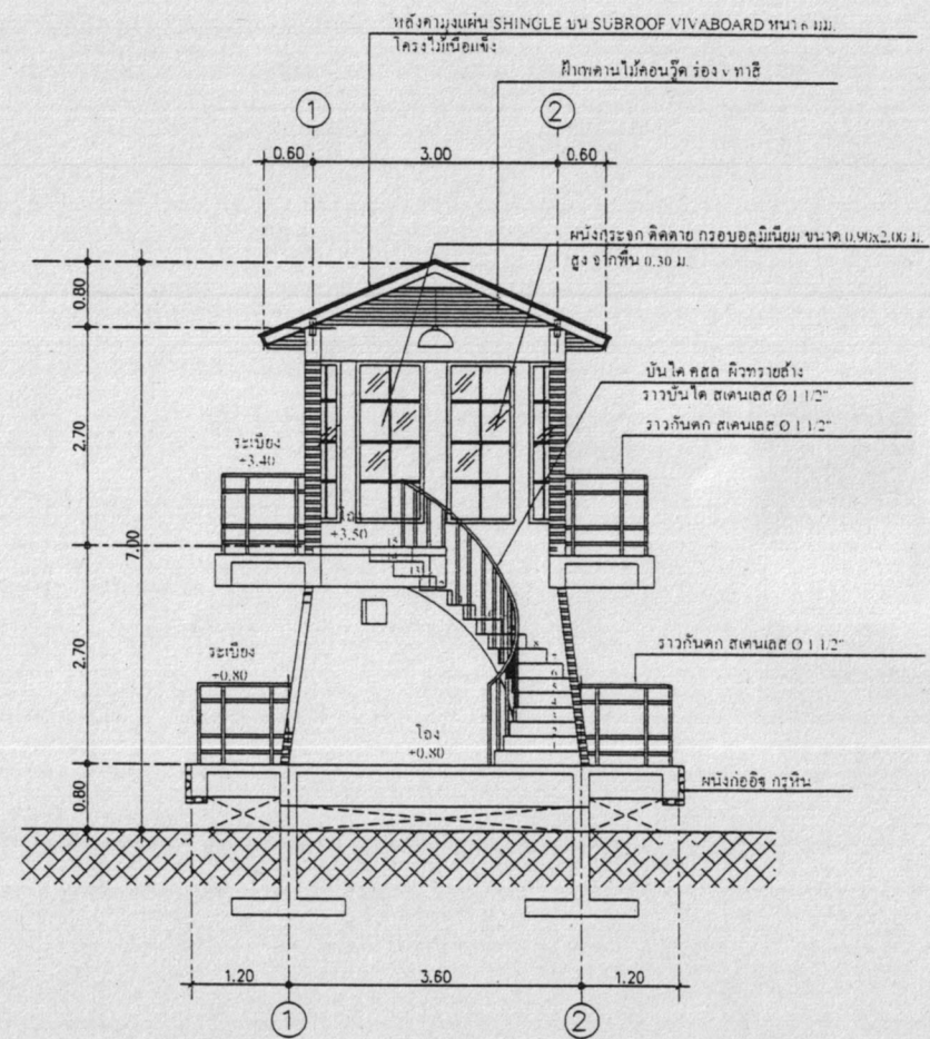
รูปตัด B SCALE 1 : 25
