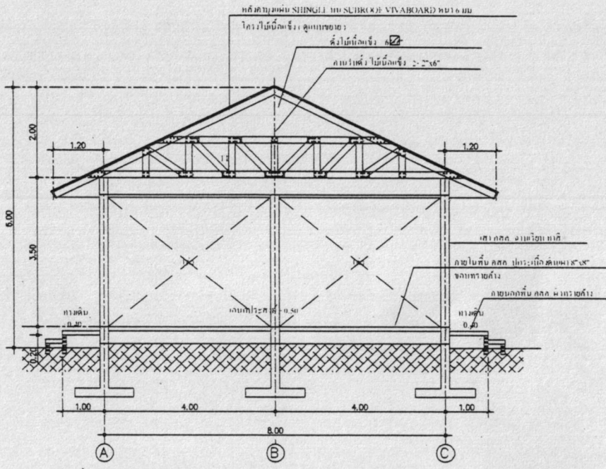
รูปตัด B SCALE 1 : 75
