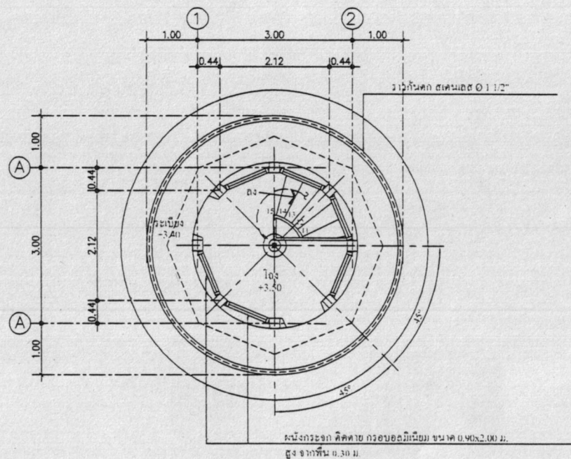
แปลนพื้นชั้นบน SCALE 1 : 75
