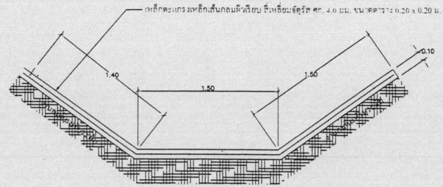
รูปตัดรางระบายน้ำรูปตัววี คสล.
