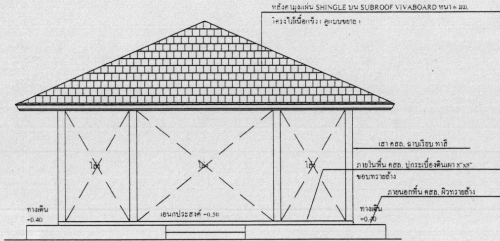
รูปด้าน 1 SCALE 1 : 75
