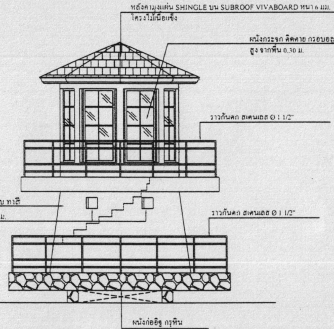
รูปด้าน 3 SCALE 1 : 75
