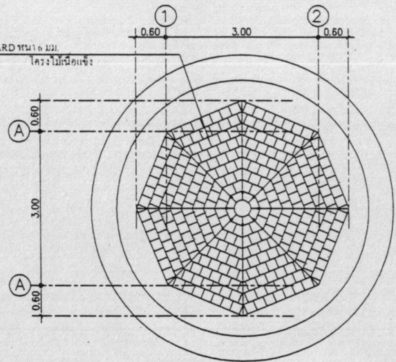
แปลนพื้นชั้นบน SCALE 1 : 75
