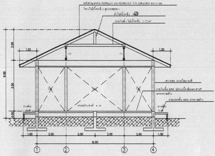
รูปตัด A SCALE 1 : 75
